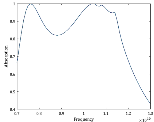
شکل (۳): نمودار جذب ساختار سلول واحد جاذب فراماده با زاویه برخورد مستقیم.
