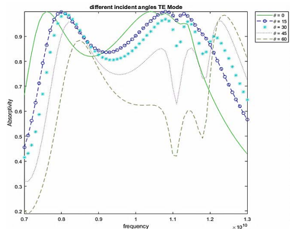
شکل (۴): نمودار جذب ساختار سلول واحد جاذب فراماده تحت زوایای تابش ۰ درجه الی ۶۰ درجه.
