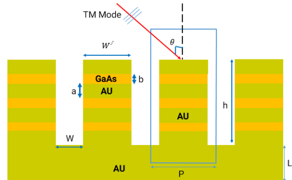
شکل (۲): شمای عرضی از نانو توری طراحی شده مرکب گالیوم آرسناید و طلا.
