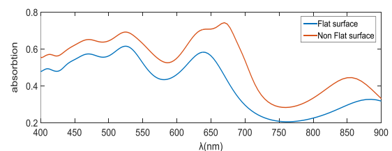
شکل (۵): نمودار طیف جذب ساختار مسطح (منحنی آبی) و غیر مسطح (منحنی قرمز) با h=200\text{ nm} .
