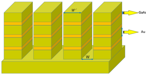
شکل (۳): شمای سه بعدی از نانو توری طراحی شده مرکب گالیوم آرسناید و طلا.
