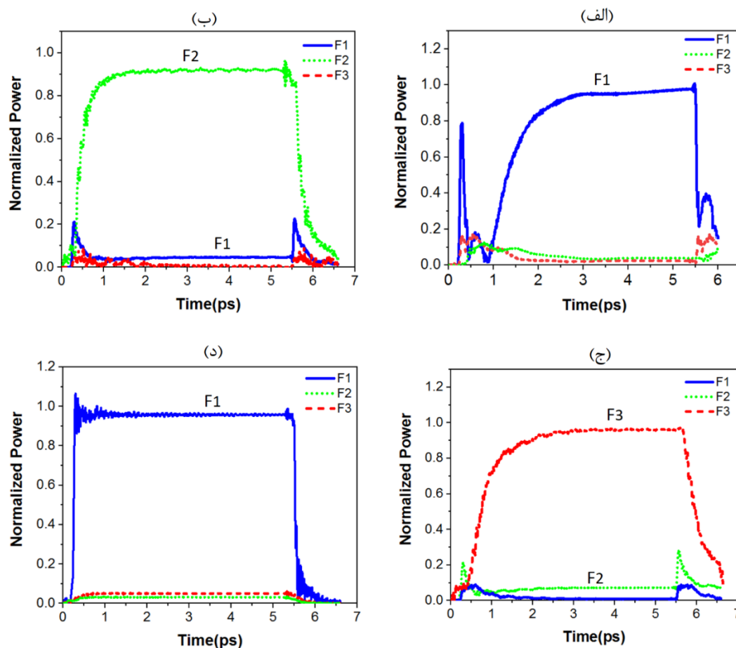
شکل (۶): توان نرمالیزه خروجی مقایسه‌کننده تک‌بیتی تمام نوری پیشنهادی برای حالت‌های (الف) X=0 و Y=0 (ب) X=0 و Y=1 (ج) X=1 و Y=0 (د) و X=1 و Y=1 که در صورت فعال بودن هر یک از ورودی‌ها، منع ورودی به صورت پالسی با عرض ۵ پیکوثانیه در نظر گرفته شده است.
