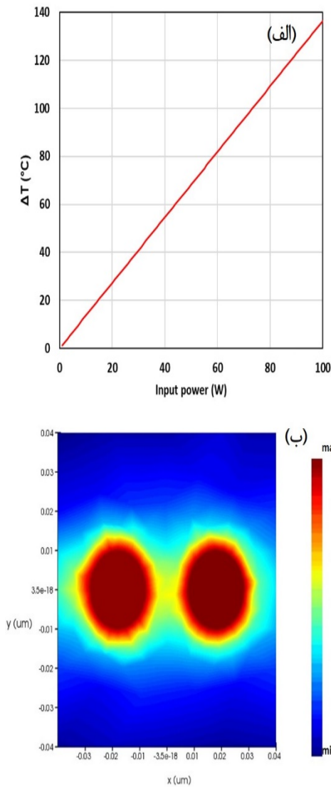
شکل (۶). (الف) نمودار افزایش دمای سطح زیرلایه نسبت به دمای اتاق (۳۰۰ درجه کلوین) بر حسب افزایش توان نور تکفام ورودی از ۱ تا ۱۰۰ وات با قطر لکه‌ی نور ۷ میلی‌متر. (ب) نمودار دمای سطح زیرلایه برای دو نانوجزیره
