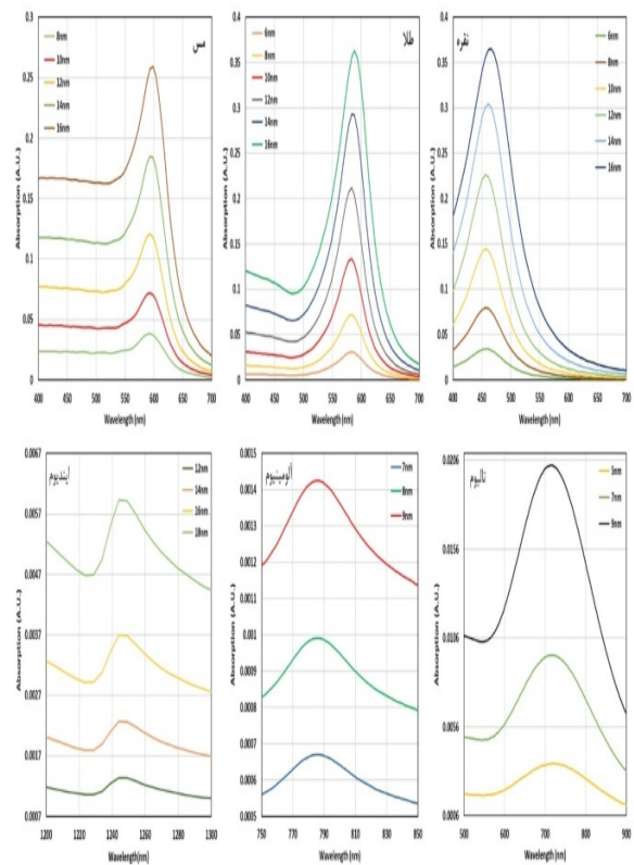
شکل (۵). شبیه‌سازی طیف جذب نانوذرات فلزی با ضخامت‌های مختلف از جنس نقره، طلا، مس، تالیوم، آلمینیوم و ایندیوم.
