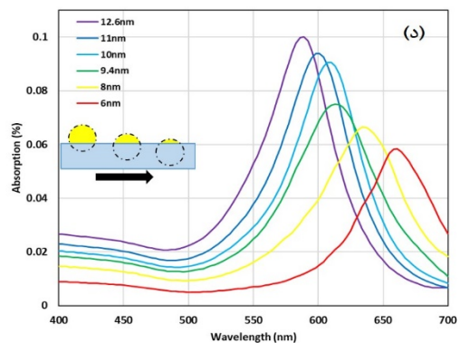
شکل (۴). شبیه‌سازی تاثیر (الف) ضریب شکست محیط، (ب) ساختار نانوجزیره، (ج) تعداد نانوجزیره شبیه‌سازی شده و (د) میزان فرورفتگی نانونیم‌کره‌های فلزی در زیر لایه بر محل جذب نانوذرات
