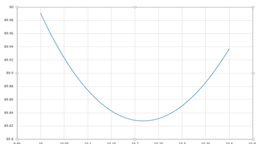
شکل (۱۱). اختلاف فاز S_{21} مود زوج و فرد
