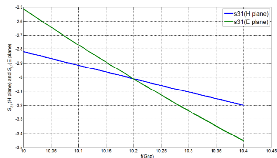
شکل (۸). مقایسه S_{31} تزویج‌گرهای صفحه E و صفحه H
