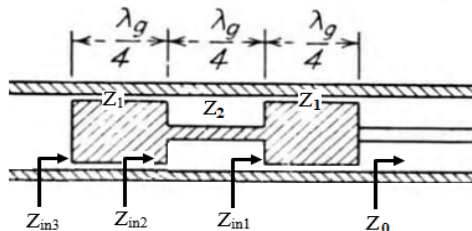
شکل (۲۲). امپدانس‌های دیده‌شده در قسمت‌های مختلف در طرح پیشنهادی (الف)
