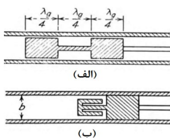
شکل (۲۱). طرح‌های پیشنهادی برای پیستون غیر اتصالی داخل موجبر
