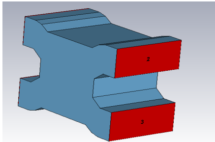
شکل (۱۷). نمای سه‌بعدی تزویج‌گر صفحه E در CST
