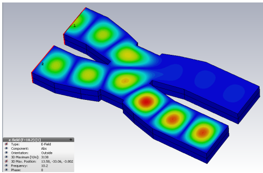
شکل (۱۶). توزیع میدان الکتریکی در تغییردهنده فاز طراحی شده در نرم‌افزار CST
