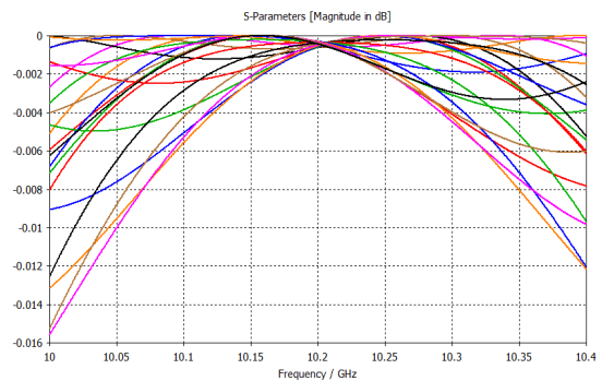
شکل (۱۴). تلفات عبوری تغییردهنده فاز صفحه H در نرم‌افزار CST برای موقعیت‌های مختلف اتصال کوتاه
