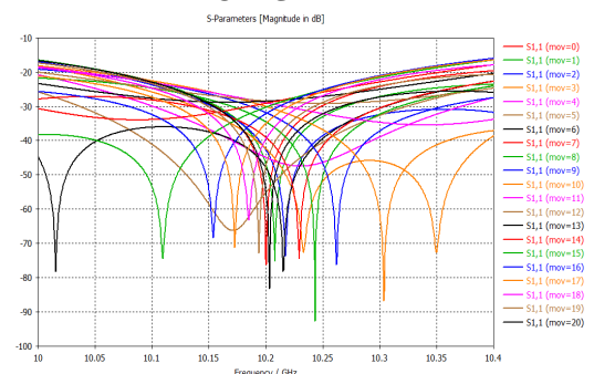
شکل (۲۰). نمودار S_{11} تغییردهنده فاز صفحه E در CST
