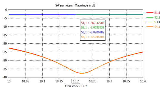
شکل (۱۹). پارامترهای پراکندگی تزویج‌گر صفحه E در CST
