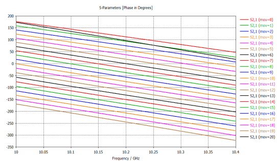
شکل (۱۵). تغییرات فاز تغییردهنده فاز صفحه H در نرم‌افزار CST
