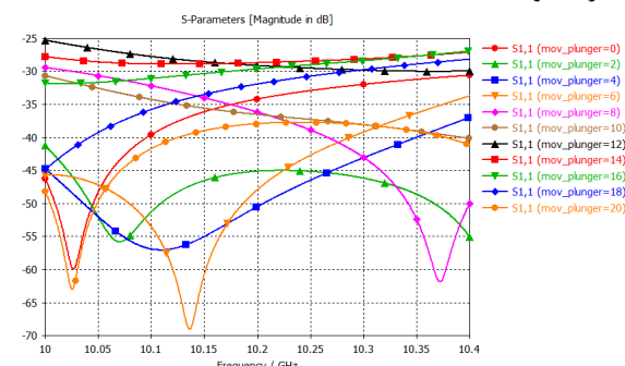
شکل (۲۶). نمودار S_{11} سیستم تغییردهنده فاز یکپارچه در CST
