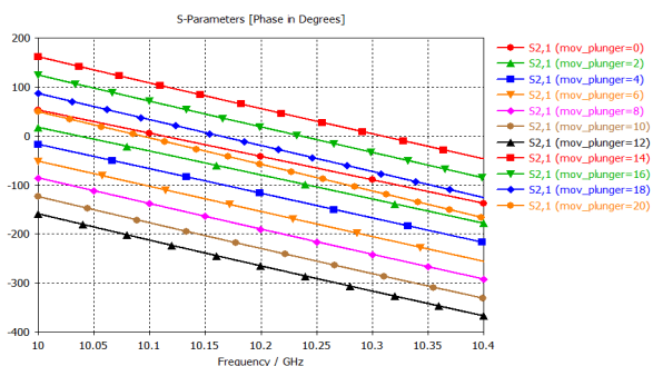
شکل (۲۵). نمودار تغییرات فاز خروجی در اثر حرکت پیستون در CST
