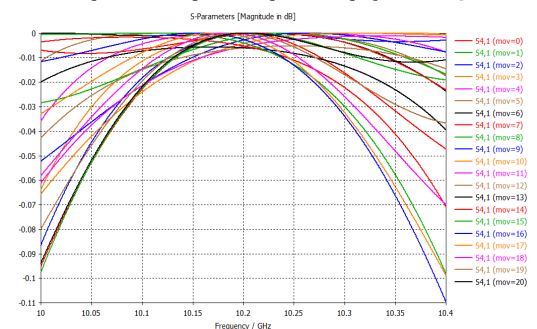
شکل (۲۵). توان عبوری تغییردهنده فاز صفحه E در CST
