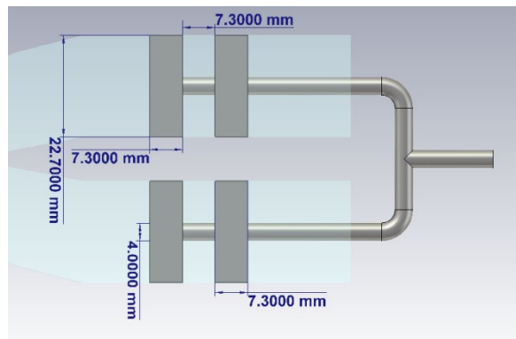
شکل (۲۳). نمایی از پیستون‌های متصل به هم در داخل ساختار
