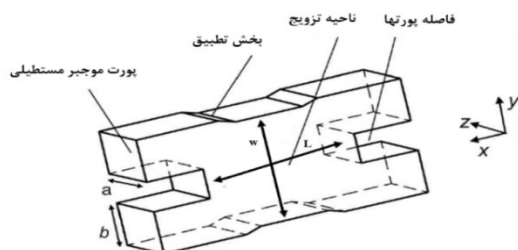
شکل (۵). شماتیک تزویج‌گر دورگه ۹۰ درجه صفحه E
