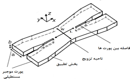
شکل (۴). شماتیک تزویج‌گر دورگه ۹۰ درجه صفحه H
