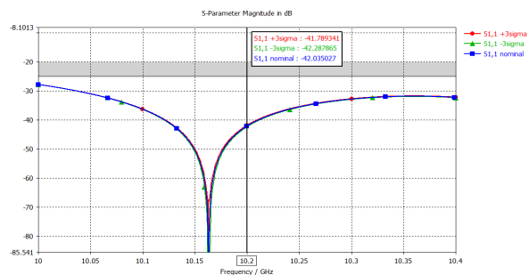
شکل (۲۹). نتایج آنالیز بهره
