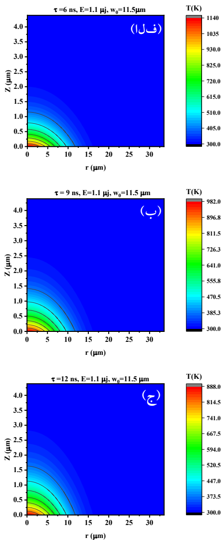
شکل (۶). نمودار توزیع فضایی دما در فلز طلا تحت تابش توسط هارمونیک دوم لیزر Nd-YAG با انرژی پالس ۱/۱ میکروژول، اندازه لکه لیزری ۱۱/۵ میکرومتر و پهنای زمانی پالس لیزری الف (۶، ب) ۹ و ج) ۱۲ نانوثانیه در زمان رسیدن پالس لیزر به بیشینه توان (۱۸ نانوثانیه).
