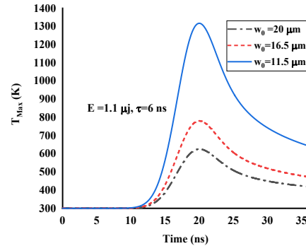
شکل (۴). نمودار تغییرات دمای طلا بر حسب زمان تحت تابش توسط هارمونیک دوم لیزر Nd-YAG با پهنای زمانی پالس ۶ نانوثانیه، انرژی پالس ۱/۱ میکروژول و شعاع‌های لکه‌ی ۱۱/۵، ۱۶/۵ و ۲۰ میکرومتر.
