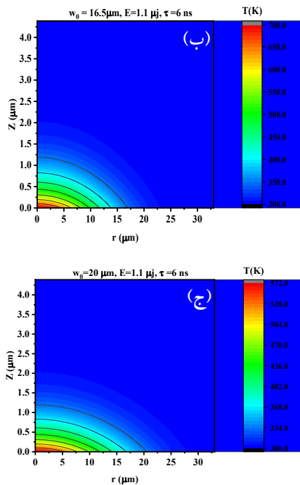
شکل (۳). توزیع دما در فلز طلا تحت تابش توسط هارمونیک دوم لیزر Nd-YAG با انرژی پالس ۱/۱ میکرو ژول، پهنای زمانی پالس ۶ نانوثانیه و شعاع لکه لیزری الف) ۱۱/۵، (ب) ۱۶/۵ و (ج) ۲۰ میکرومتر در زمان ۱۸ نانوثانیه.
