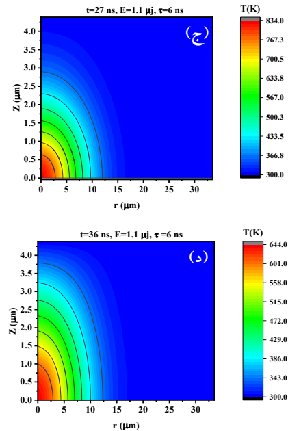
شکل (۲). توزیع دما در فلز طلا تحت تابش توسط هارمونیک دوم لیزر Nd-YAG با انرژی پالس ۱/۱ میکروژول، پهنای زمانی پالس ۶ نانوثانیه و اندازه لکه لیزری الف) ۱۱/۵ میکرومتر در زمان های الف) ۹، (ب) ۱۸، (ج) ۲۷، (د) ۳۶ نانوثانیه.
