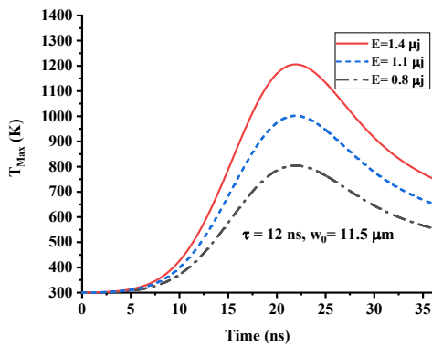
شکل (۵). نمودار تحول زمانی دمای بیشینه طلا تحت تابش توسط هارمونیک دوم لیزر Nd-YAG با پهنای زمانی پالس ۱۲ نانوثانیه، شعاع لکه ی ۱۱/۵ میکرومتر و انرژی‌های پالس مختلف.
