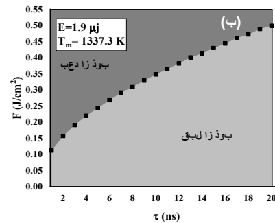
شکل (۸). الف، نمودار آستانه‌ی ذوب طلا تحت تابش توسط
